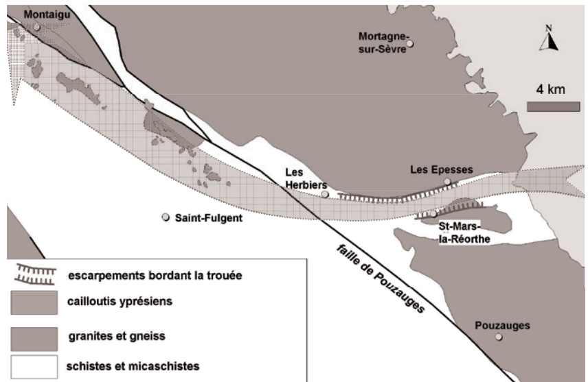
▲ Carte géologique simplifiée de la région des Herbiers et tracé supposé du fleuve yprésien
